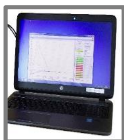
Logiciel InSiTox 1.0
